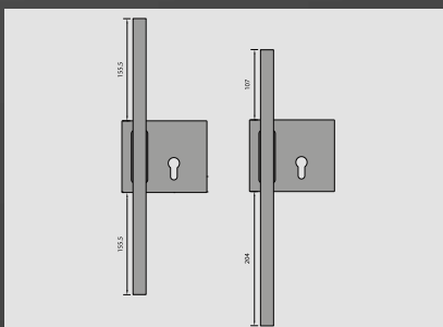
Griffstangen für Schiebetürschloss Tvin 2.0: G 420 rund oder G420 eckig/breit
